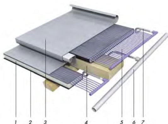
Abb. 7: Unverglaster Sonnenkollektor QUICK STEP®-SolarThermie
